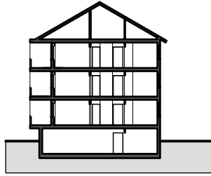
Schnitt
